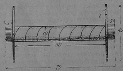
Рис. 2. Катушка.
