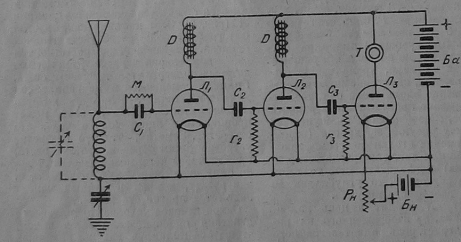
Рис. 1. Схема усилителя.
