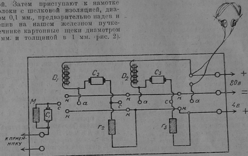
Рис. 3. Монтажная схема.
