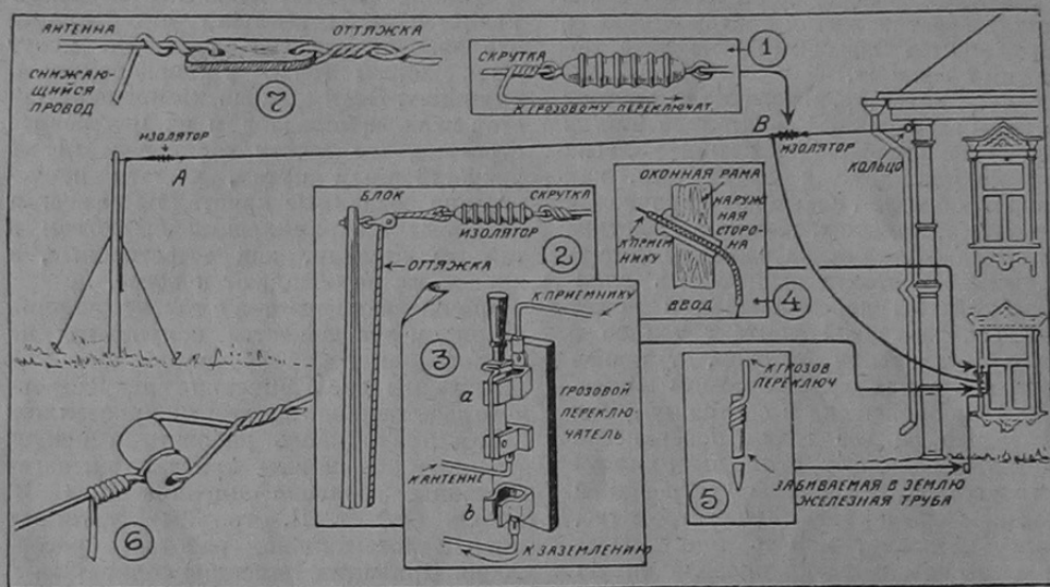
Любительская антенна и ее детали:
