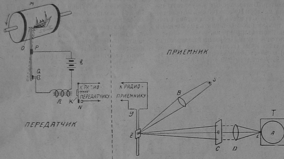
Рис. 3. Схема работы аппарата Белена.
